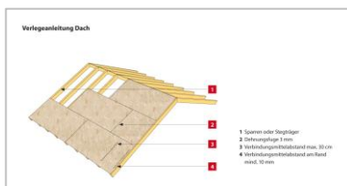
Uputstvo upotrebe SWISS KRONO OSB/3 bright ploča kod krovnih konstrukcija (Izvor slika: INTERSPAN Faipari Kft.)
