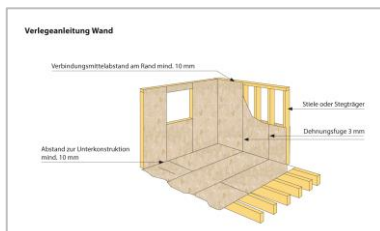
Uputstvo upotrebe SWISS KRONO OSB/3 bright ploča kod zidnih konstrukcija (Izvor slika: INTERSPAN Faipari Kft.)
