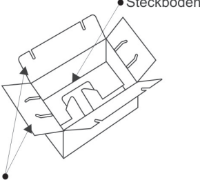
Mit QUICK Lock Deckelschnellverschluss
