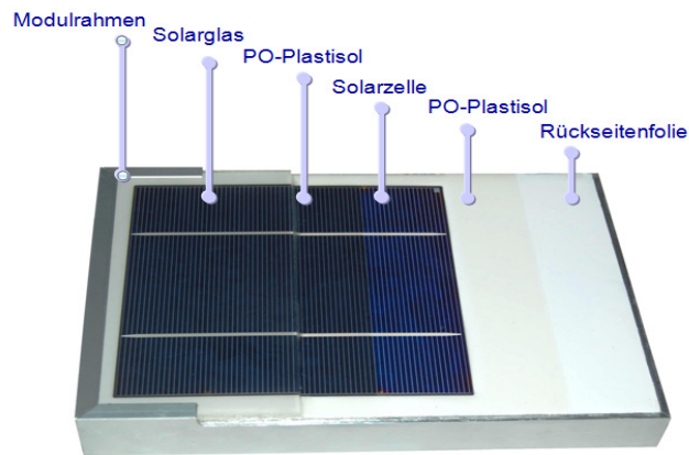
Abb. 4 Schichtaufbau eines Solarmoduls
