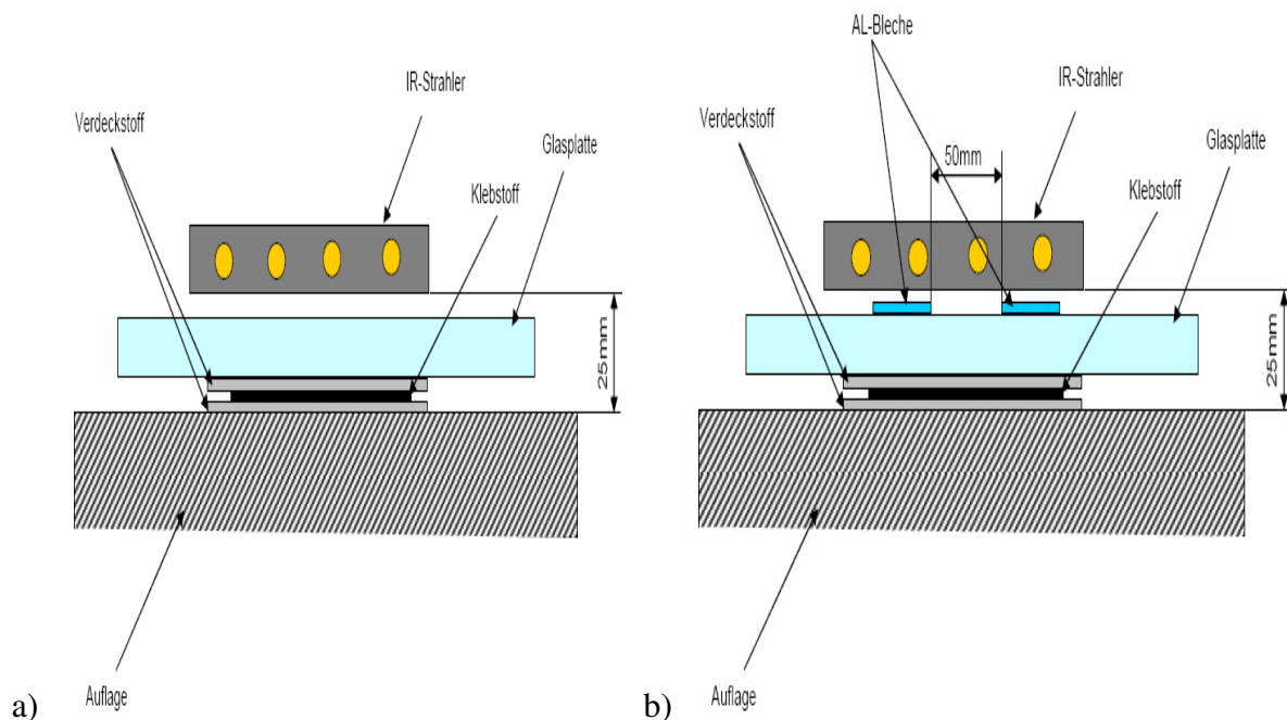
Abb. 3 Verklebung von Textil durch a) Glasplatte unter STIR®
