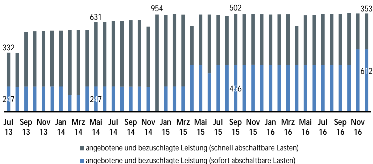
Abbildung 66: Im Zeitraum von Juli 2013 bis Dezember 2016 ausgeschriebene und bezuschlagte Abschaltleistung getrennt nach sofort und schnell abschaltbaren Lasten.
