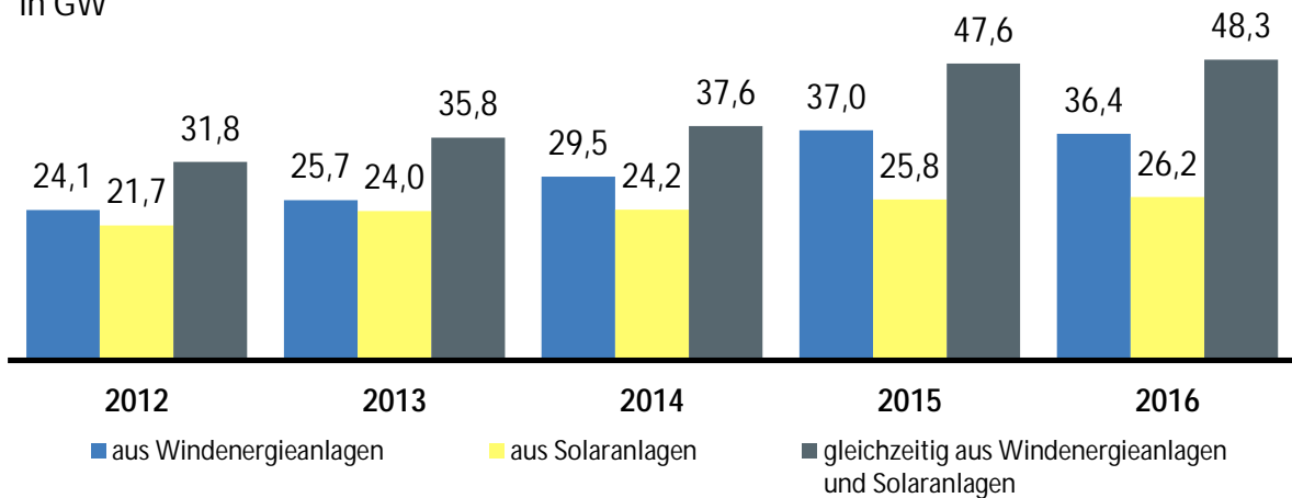
Abbildung 16: Maximale Einspeisung
