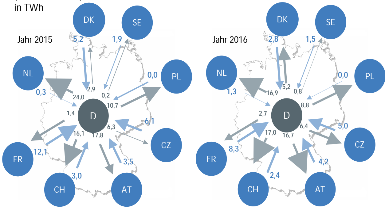
Abbildung 69: Physikalische Lastflüsse
